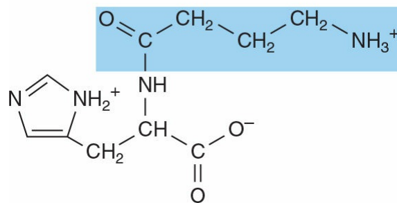
Homocarnosine
