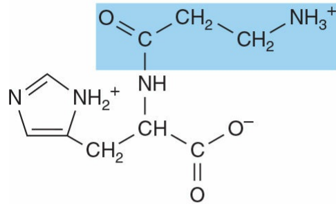
Carnosine
