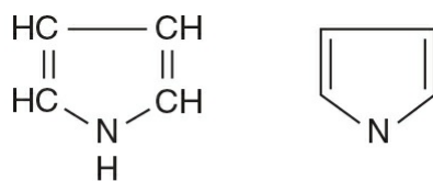
Pyrrole
