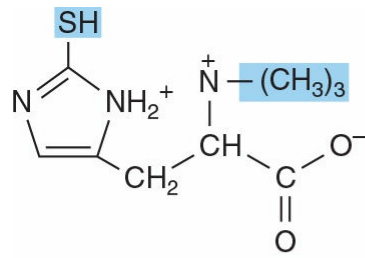
Ergothioneine
